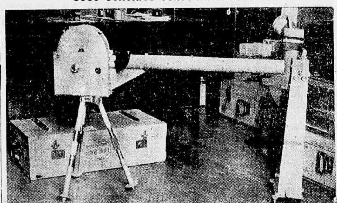
O sismographo de refração: um dos instrumentos que demonstraram a pequena amplitude dos movimentos de terra em Bomsucesso
